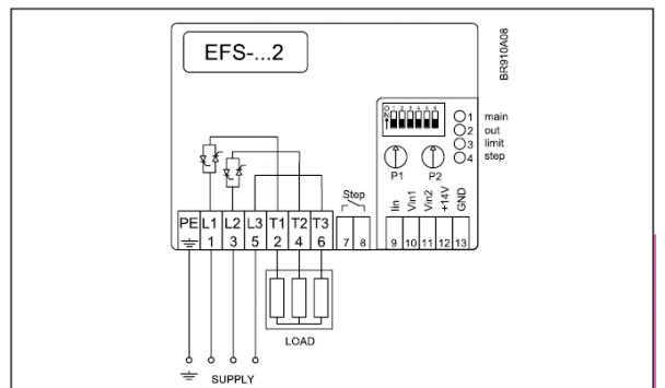
Obciążenie symetryczne (podłączenie w gwiazdę)
