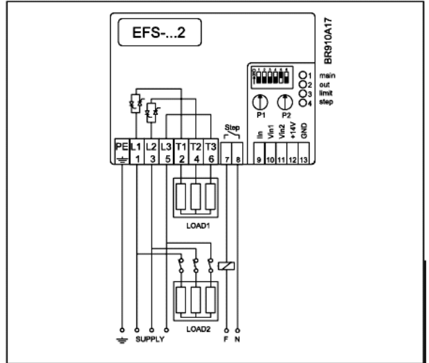
Fig 1 Podwojenie mocy wyjściowej z wykorzystaniem wewnętrznego przełącznika.
